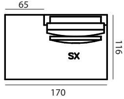
LATERALE TERMINALE DEEP DX / SX
